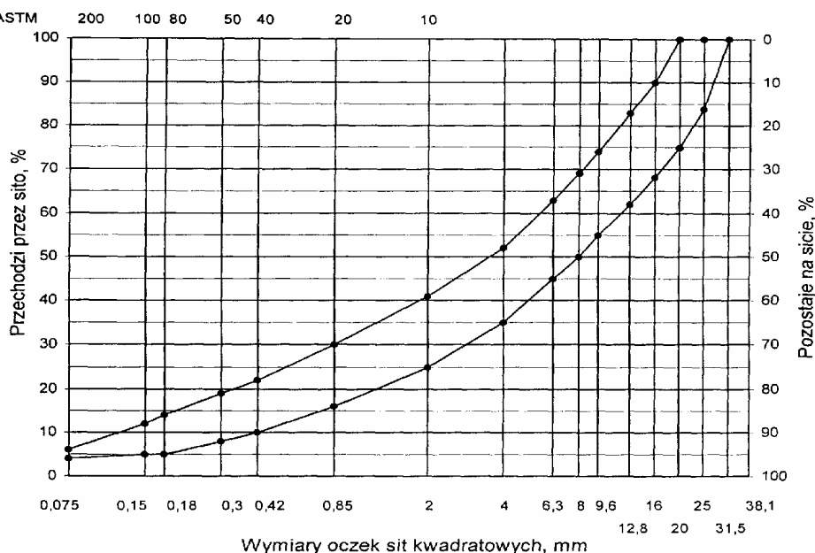
Rys. 11. Krzywe graniczne uziarnienia mieszanki mineralnej BA od 0 do 25 mm do warstwy wiążącej, wyrównawczej i wzmacniającej
