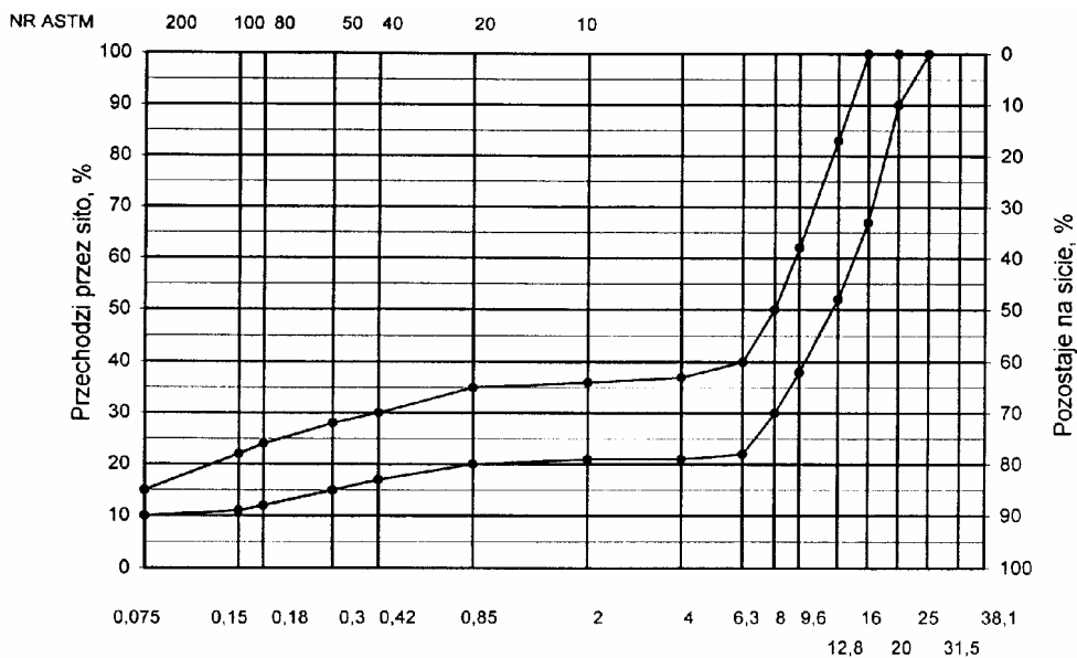
ys. 5. Krzywe graniczne uziarnienia mieszanki mineralnej BA od 0 do 20 mm (mieszanka o nieciągłym uziarnieniu) do warstwy ścieralnej nawierzchni drogi o obciążeniu ruchem od KR3 do KR6
